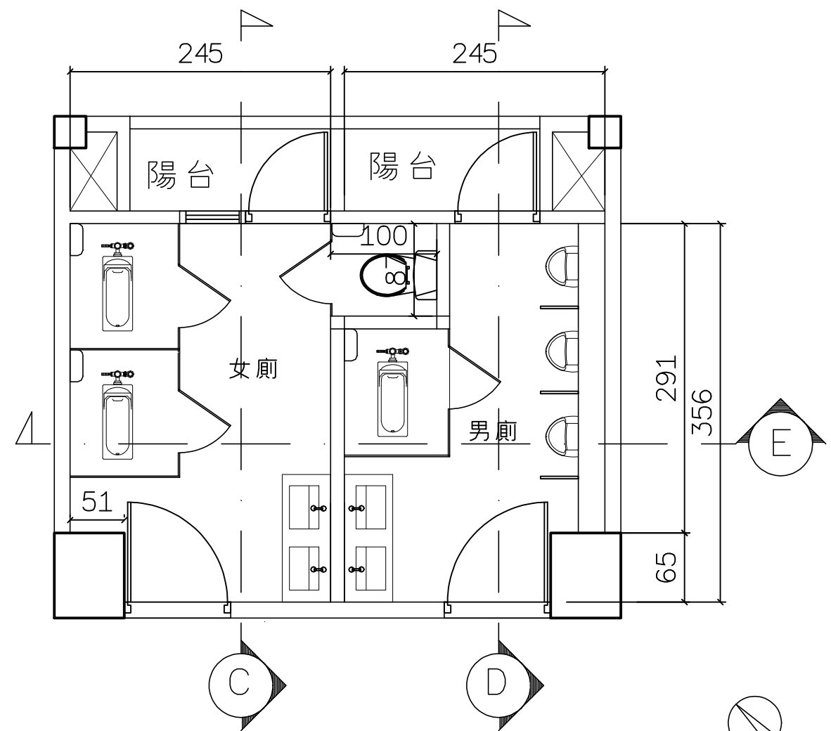
二~四層廁所平面配置圖
