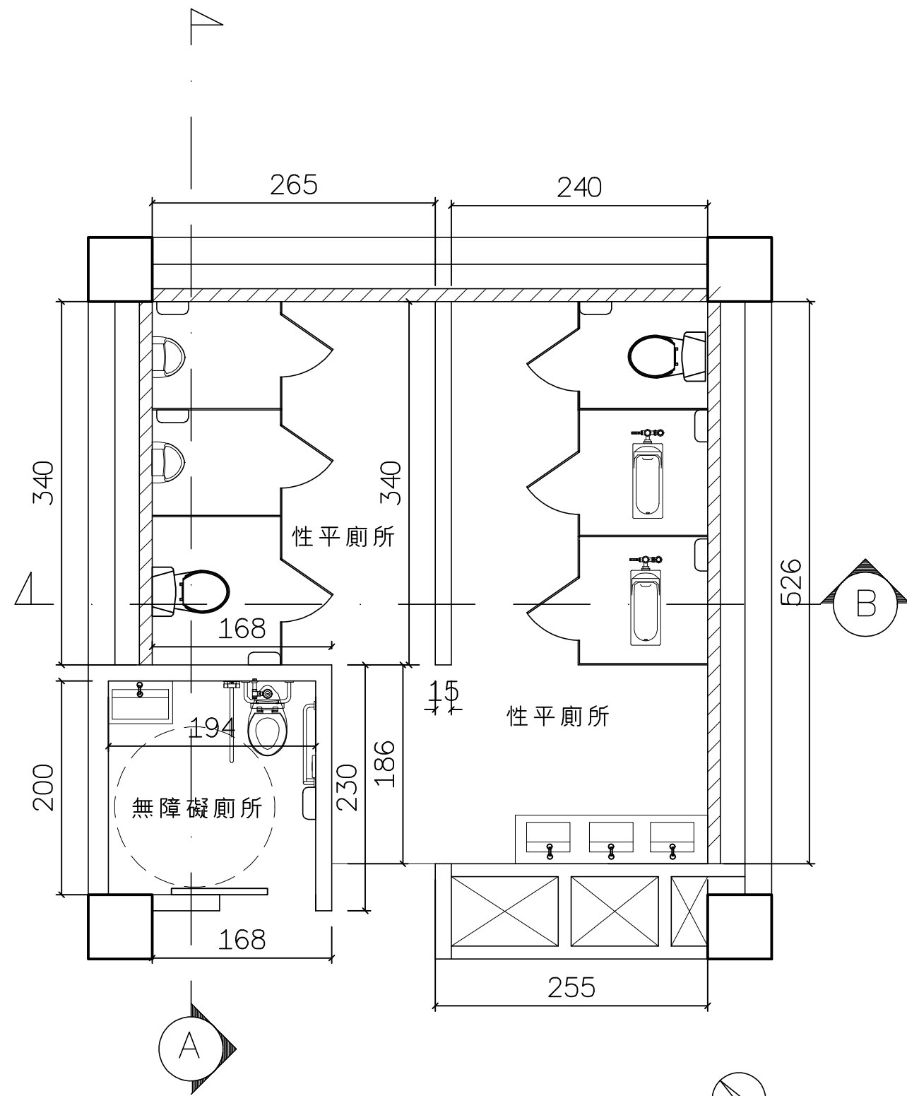
地下一層廁所平面配置圖
