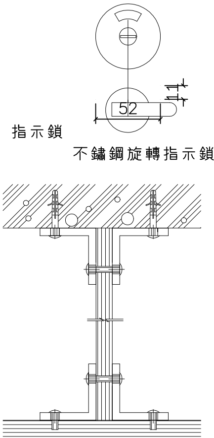
角鐵安裝剖面圖
